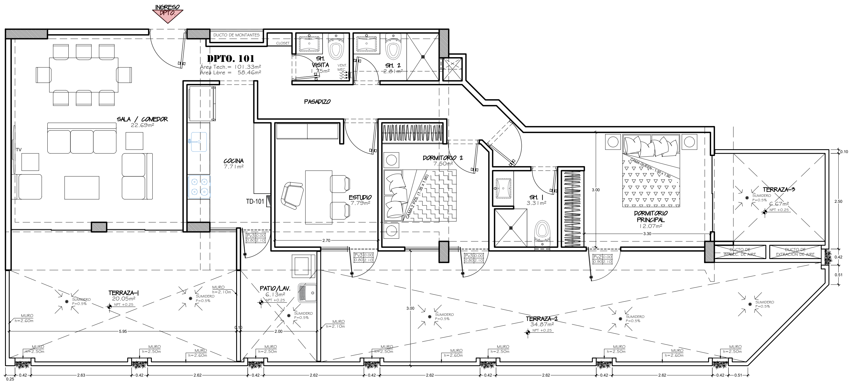
PLANTA DPTO. FLAT 101
